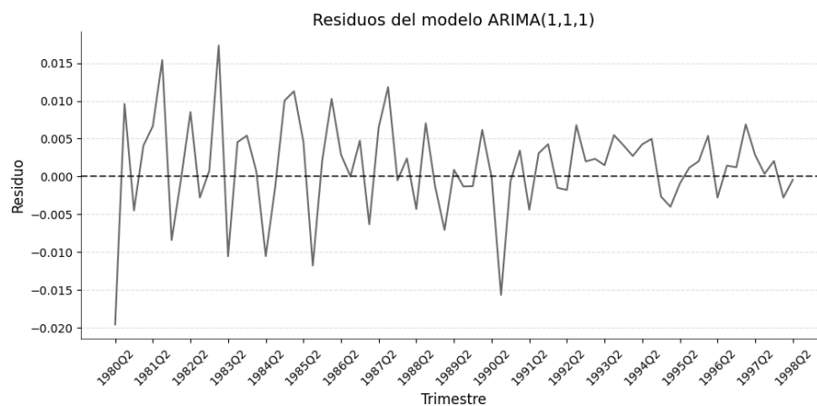
Figura 13: Residuos de estimación del modelo ARIMA(1,1,1)
